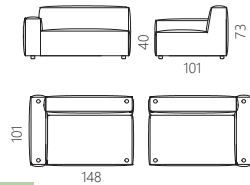
ID : 3009-43F 3009-44F 1-arm wide/LHF 1-arm wide/RHF
